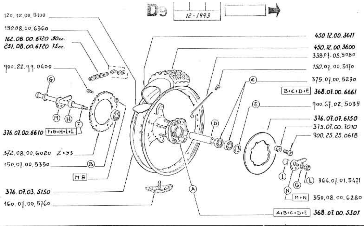
376.07.07.5290 Ruota post. completa Roue arrière complète Rear wheel complete Hinterrad Komplet
