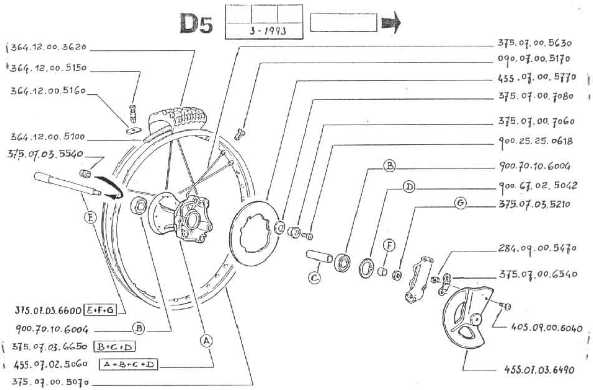
455.07.03.5000 Ruota ant. cpl. Roue avant complete Front wheel complete Vorderrad Komplett
