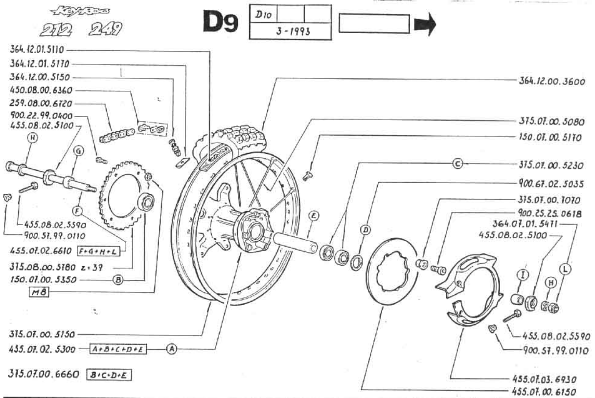
455.07.02.5290 Ruota post. cpl. Roue arriere complete Rear wheel complete Hinterrad Komplett
