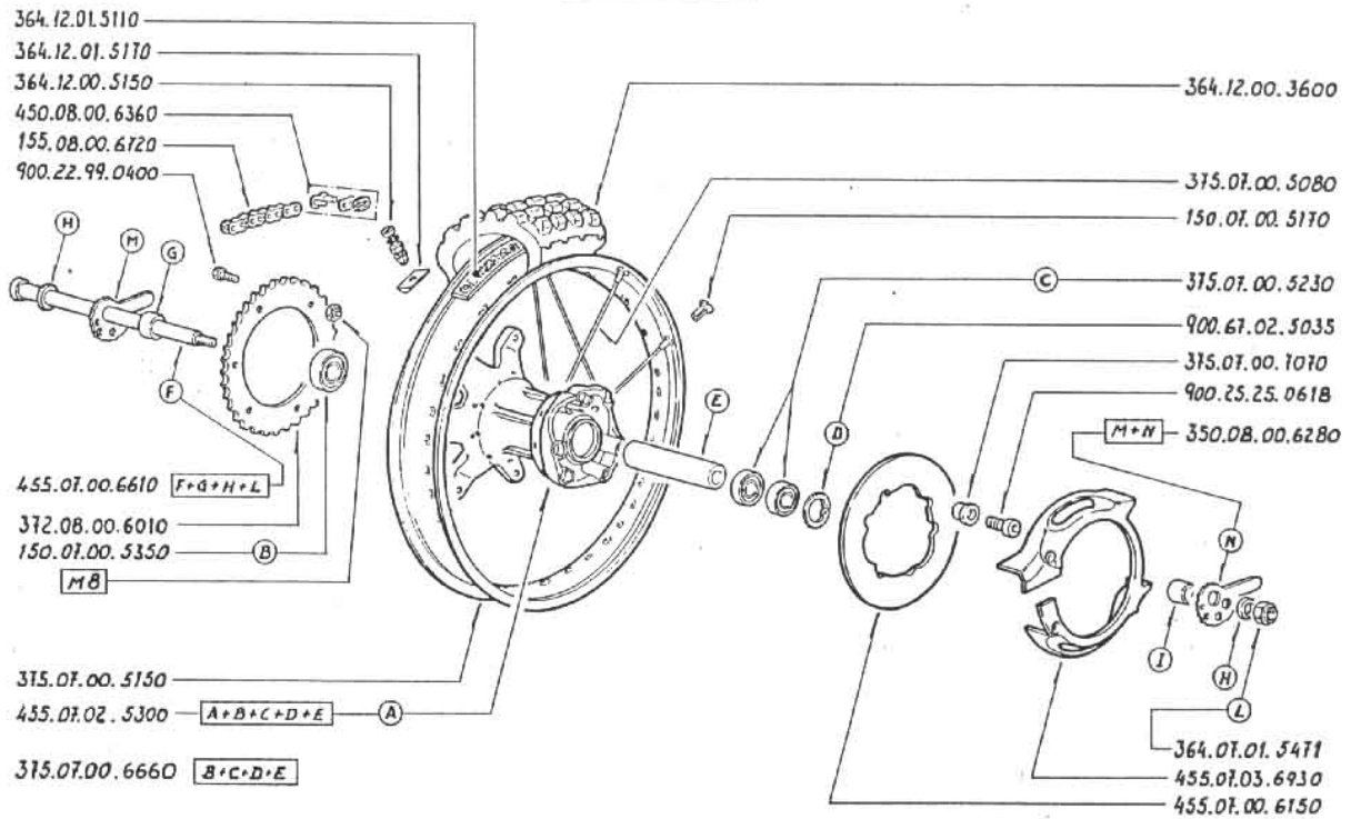
452.07.00.5290 Ruota post. cpl. Roue arriere complete Rear wheel complete Hinterrad komplett
