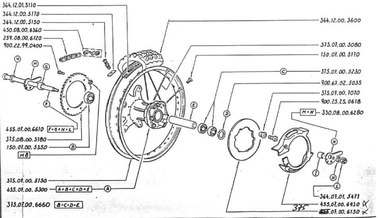
455.07.00.5290 Ruota post. cpl. Roue arriere complete Rear wheel complete Hinterrad Komplett.
