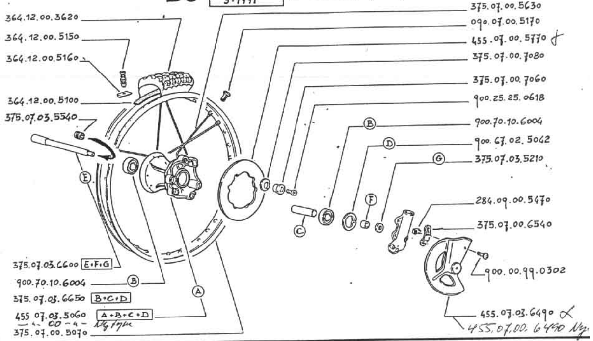
455.07.00.5000 Ruota ant. cpl. Roue avant complete Front wheel complete Vorderrad Komplett
